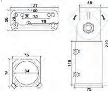
POLE CLAMP
